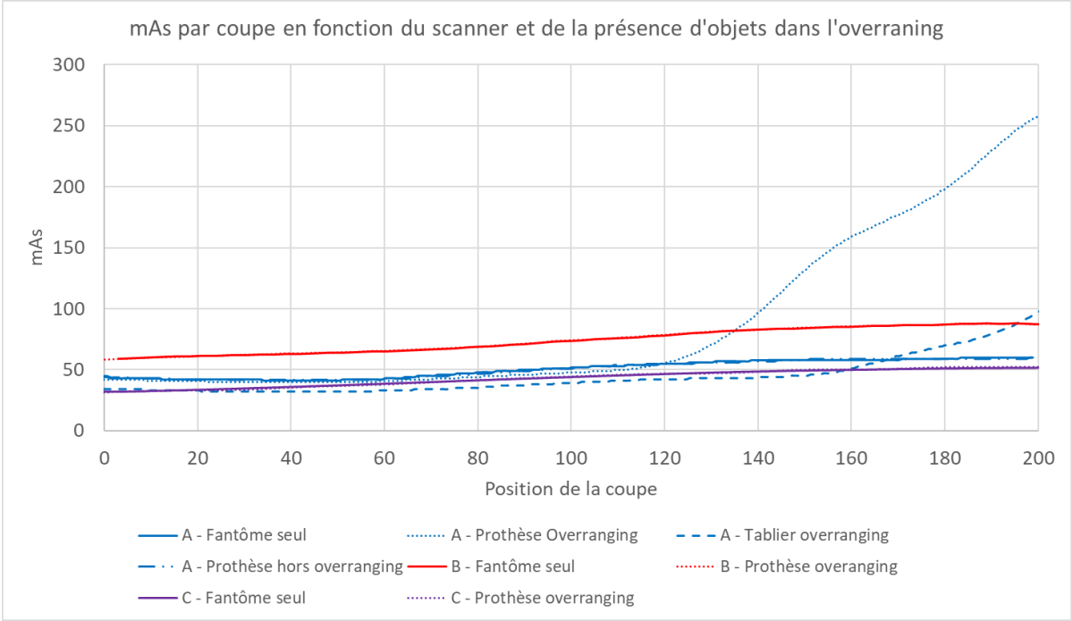
Image 2 : Graphique des mAs par coupe pour les acquisitions réalisées sur les scanners A, B et C
